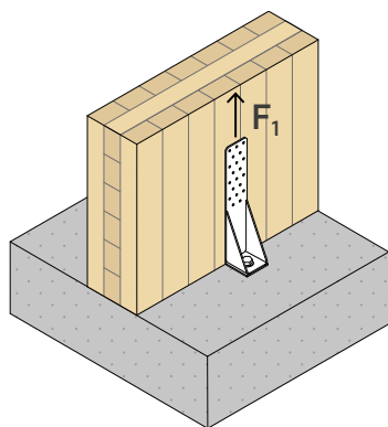
RÉSISTANCES CÔTÉ BOIS | WIDE PATTERN | fixation totale
