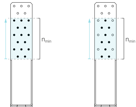
WHT20: fissaggio parziale in configurazione rispettivamente wide pattern e narrow pattern, con installazione del numero minimo di connettori n_{\min} .
