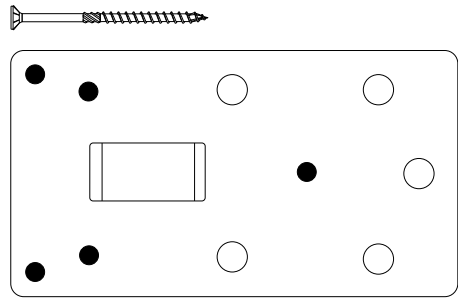
5x agujeros avellanados Ø11 mm
