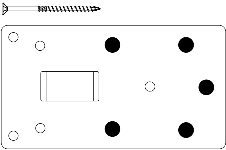
5x agujeros cilíndricos Ø13 mm
