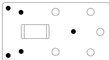
5x fori svasati Ø11 mm
