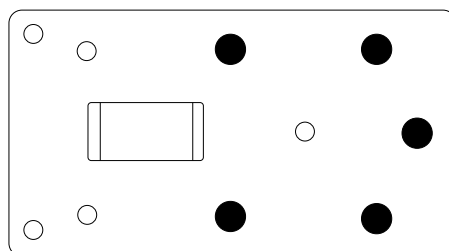
5x fori cilindrici Ø13 mm
