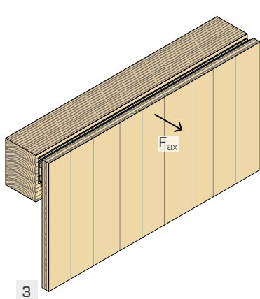
nosník | fasáda CLT
