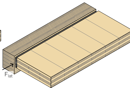
Träger | BSP-Decke
