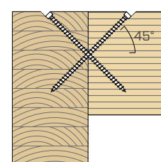
nárys
