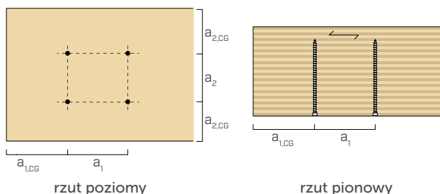
rzut poziomy
