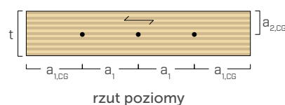
rzut poziomy
